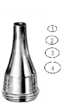
GRUBER (for adults) 44.0024.00 set/4 44.0024.01 4.5mm Ø, Fig. 1 44.0024.02 5.5mm Ø, Fig. 2 44.0024.03 6.5mm Ø, Fig. 3 44.0024.04 7.5mm Ø, Fig. 4
